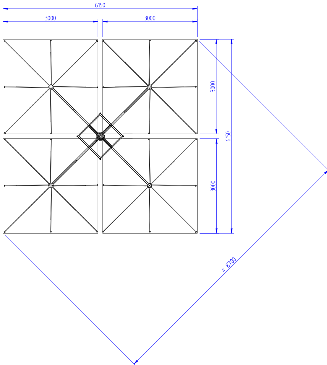
Multipole XL 300x300 QUATTRO
